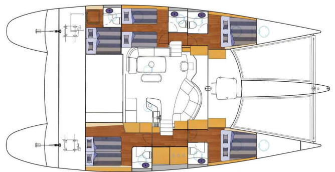
Plan intérieur cabines
